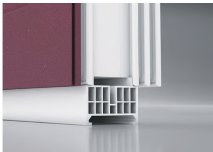
Listwa transportowo-montażowa
