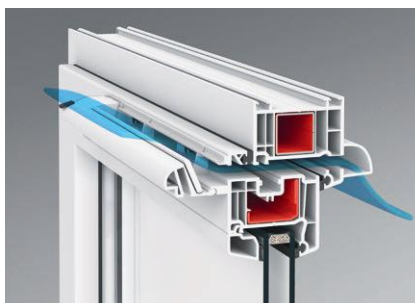
Nawiewnik higrosterowany Aereco EMM
